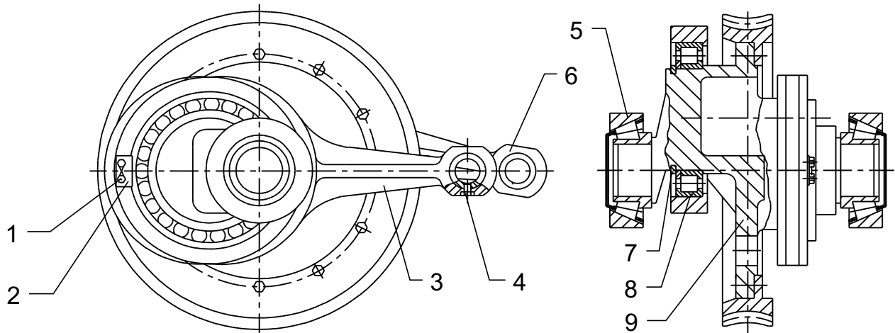
Рисунок 3 - Вал эксцентриковый с шатунами АФНИ.303141.004
