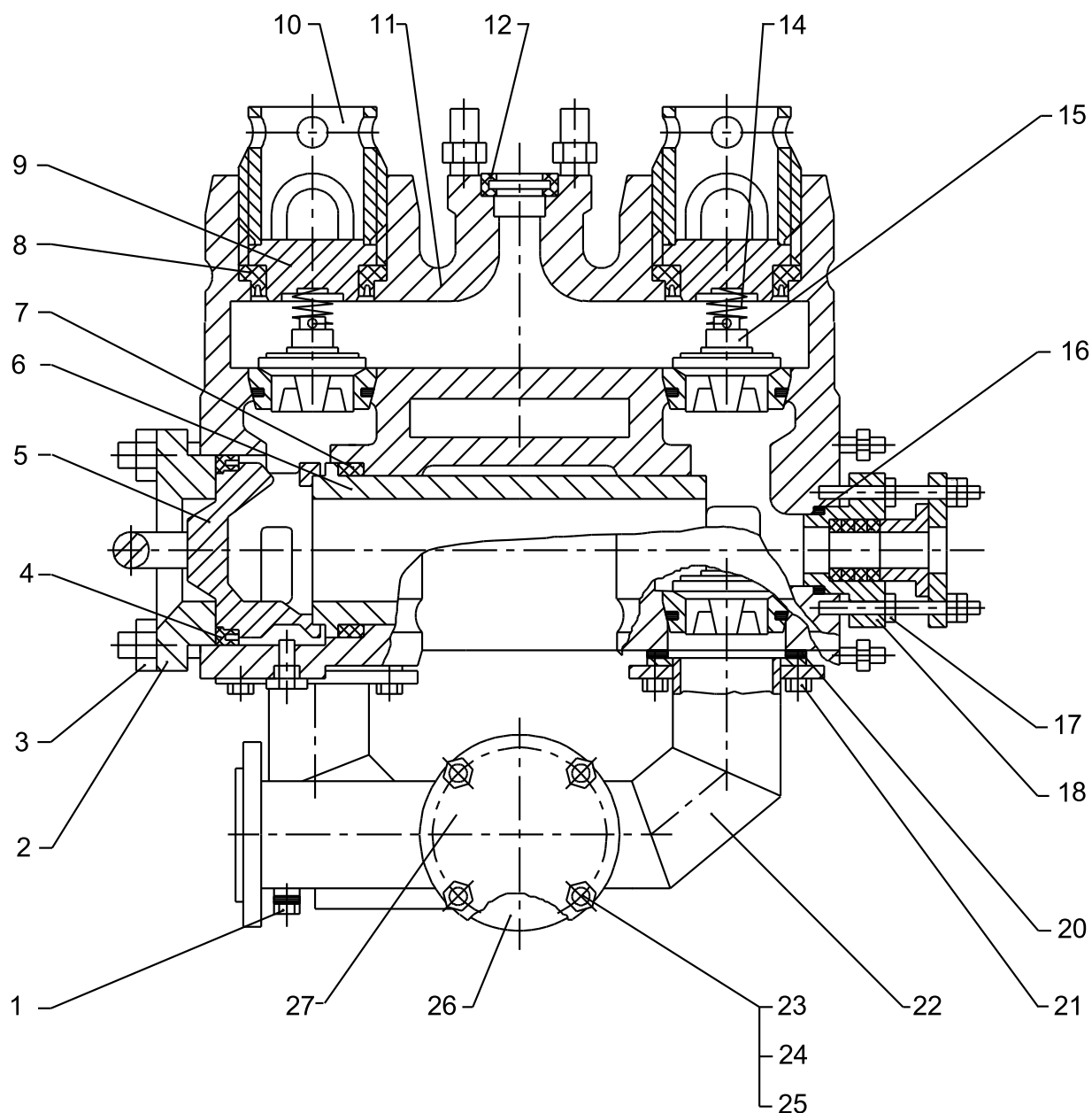
Рисунок 4 - Гидравлическая часть АФНИ.306555.001-01
