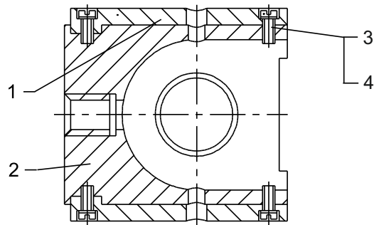
Рисунок 7 - Крейцкопф АФНИ.304516.001
