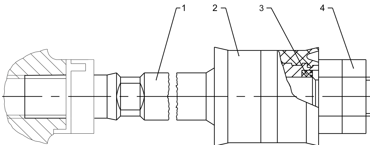
Рисунок 9 - Шток поршня с поршнем и гайками
